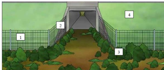
1: Malla perimetral; 2: Malla continua; 3: Vegetación natural; 4: Terraplén
